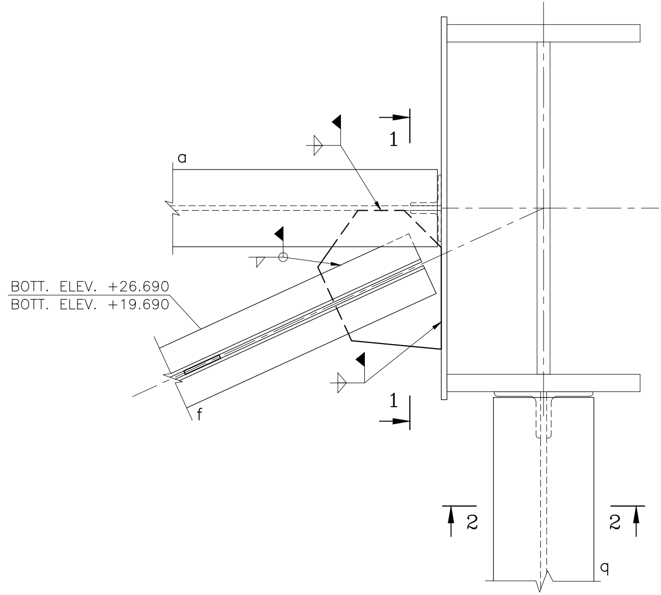
DET. "11" SS005 SC. 1:10 SS007
