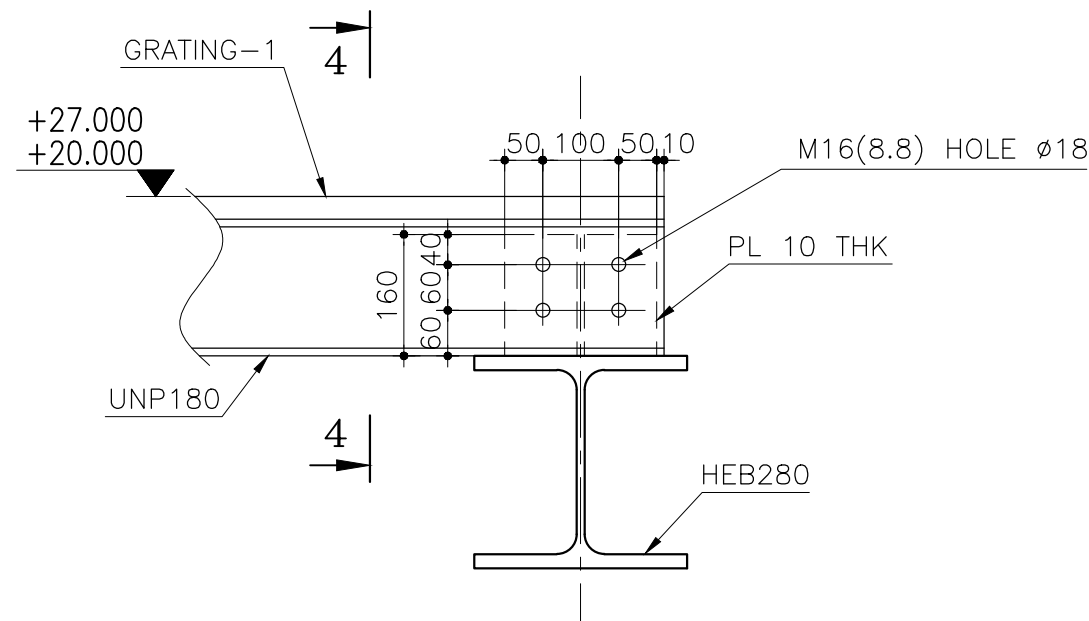
DET. "25" SS006 SC. 1:10 SS008
