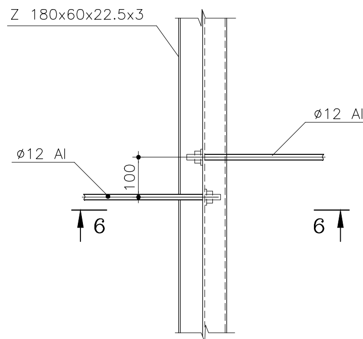
DET. "29" Sc. 1:10
