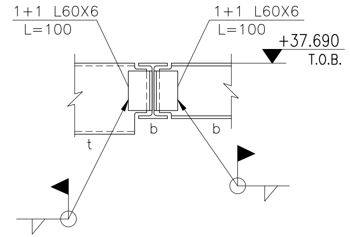
DET. "17" SC. 1:10
