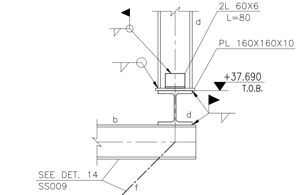
DET. "18" SC. 1:10
