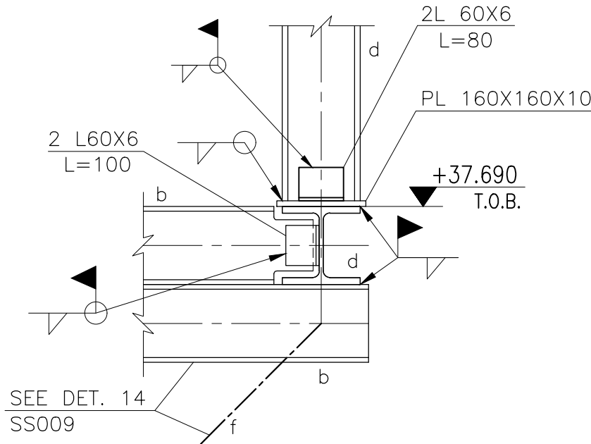
DET. "19" SC. 1:10
