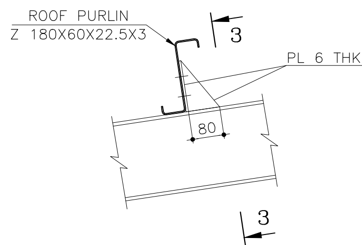
DET. "26" Sc. 1:10
