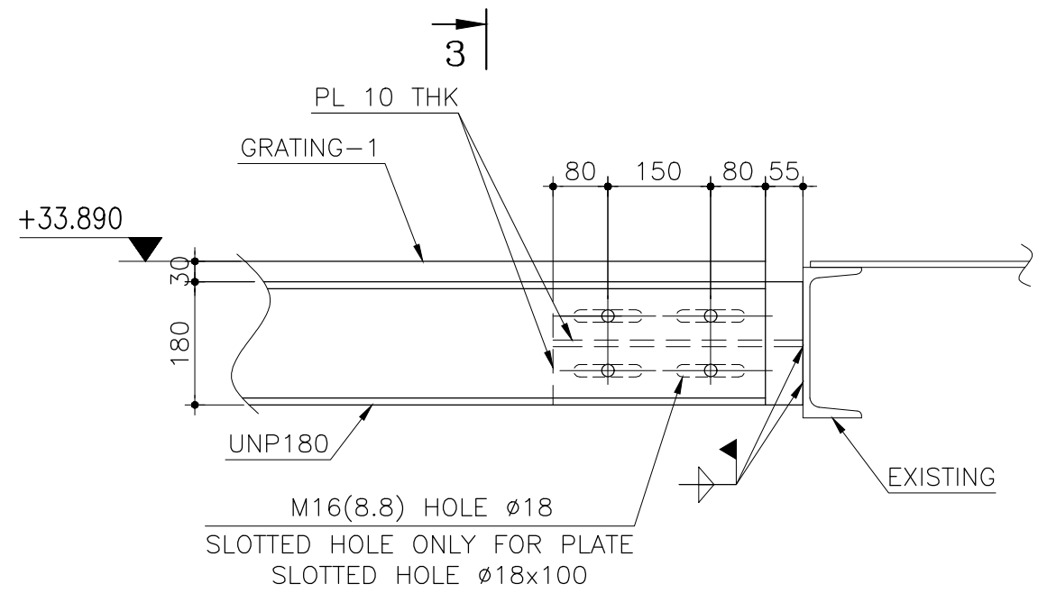
DET. "24" SS010 SC. 1:10
