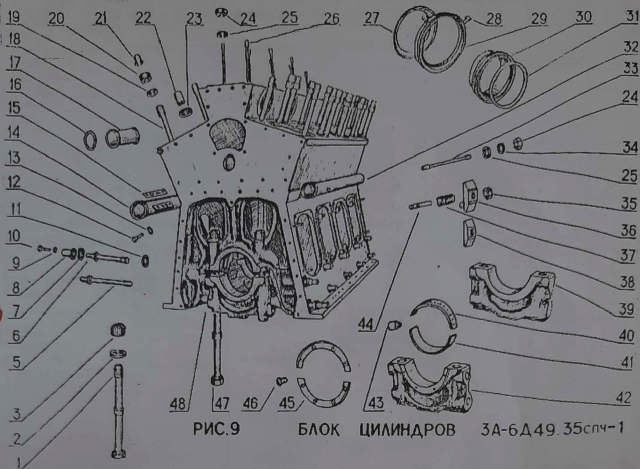
Блок цилиндров 3А-6Д49.35спч-1 Fig.9 Cylinder Block 3А-6Д49.35спч-1
